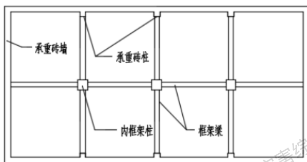
内框架结构
